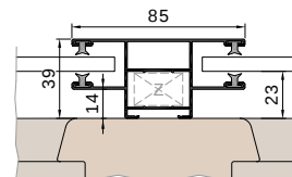
Kämpfer mit Führungs- schiene KE85V
