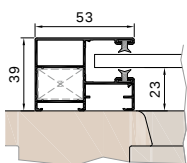
Führungsschiene KF53V
