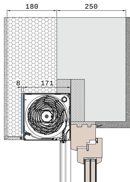
Mit Wärmedämmverbundsystem. VORO WDV.
