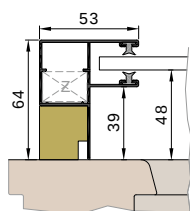
Thermisch getrennte Führungsschiene K53VT
