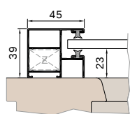
Führungsschiene KF45V
