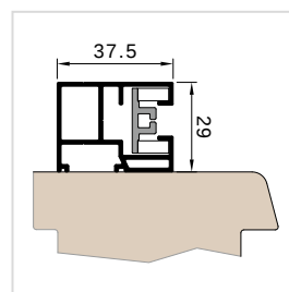
Führungsschiene FS Z37V
