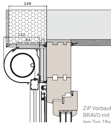
ZIP VorbauKasten BRAVO mit Endleis- ten-Typ 18x44
