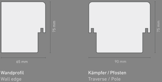
Aufbau Blockrahmen Block frame construction
