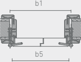
Horizontalschnitt Zarge mit Rundkante 2-flügelig gefälzte Türen
