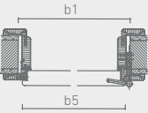
Horizontalschnitt Zarge mit Rundkante 1-flügelig gefälzte Türen
