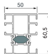
Verbreiterungsprofil VP 50
